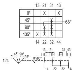
Schéma de fonctionnement 8008/-124
