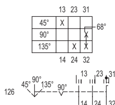
Schéma de fonctionnement 8008/-126
