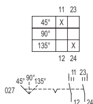
Schéma de fonctionnement 8008/-027
