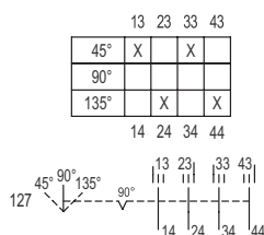
Schéma de fonctionnement 8008/-127
