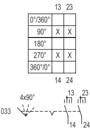
Schéma de fonctionnement 8008/2-033 Schéma de fonctionnement 8008/4-10-33
