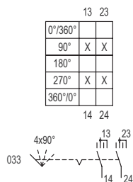
Schéma de fonctionnement 8008/-033
