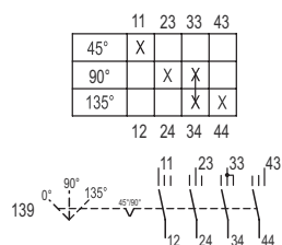
Schéma de fonctionnement 8008/-139
