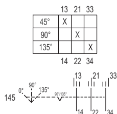
Schéma de fonctionnement 8008/-145
