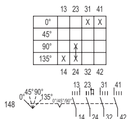
Schéma de fonctionnement 8008/-148
