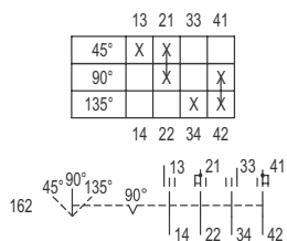
Schéma de fonctionnement 8008/-162
