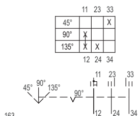
Schéma de fonctionnement 8008/-163
