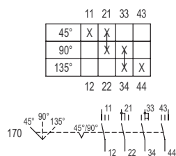
Schéma de fonctionnement 8008/-170
