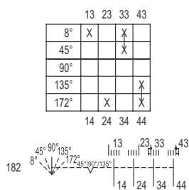
Schéma de fonctionnement 8008/-182
