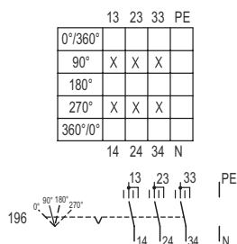
Schéma de fonctionnement 8008/-196
