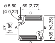
8118/1. Boîtier taille 1
