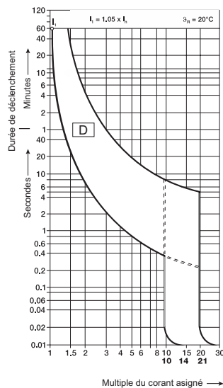
Caractéristique de déclenchement D
