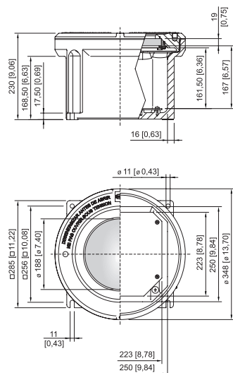
Boîtier taille 5 avec hublot
