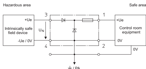
Barrières de détection un canal pour potentiel positif
