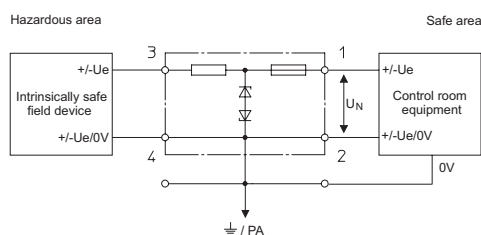
Barrières Zener de sécurité intrinsèque un canal pour potentiel variable
