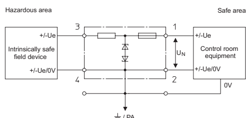
Barrières Zener de sécurité intrinsèque un canal pour potentiel variable
