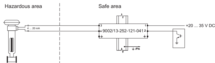
Cas d'application : sortie analogique (source de courant) pour transformateurs i/p, etc. ; circuit de terrain non mis à la terre
