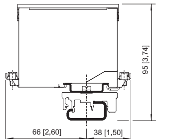
Installation sur support rail DIN NS 32 avec adaptateur et base de bride en matière moulée
