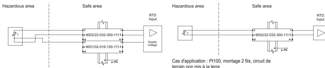
Cas d'application : Pt100, montage 3 fils, circuit de terrain non mis à la terre
