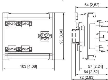
Coupleur d'appareils de terrain, 4 spurs, sans boîtier
