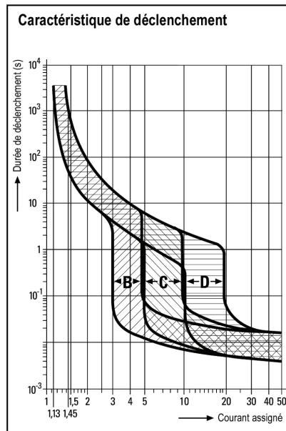
Courant général +/-, 2 pôles
