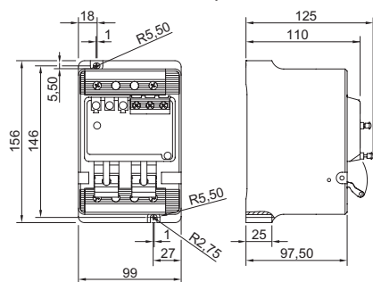
8562/54-....., 2 pôles avec contact auxiliaire et fonction de réinitialisation
