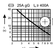
Plage de réglage : 5,5 - 8,0 A
