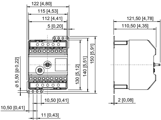
8523/82 Disjoncteur moteur Taille 2, avec contacts auxiliaires
