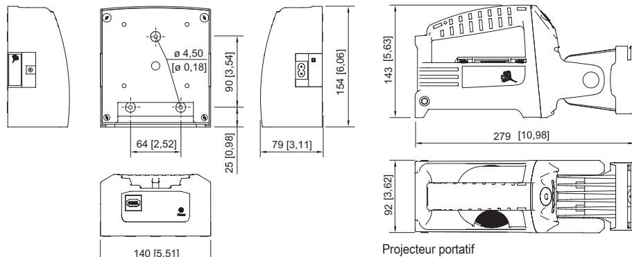
Support chargeur
