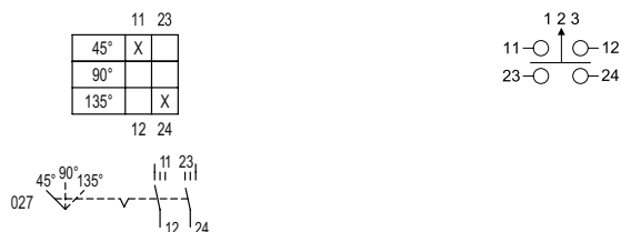
Schéma de fonctionnement 8008/-027
