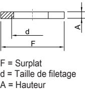
Plan d'encombrement (toutes les dimensions sont en mm [pouces]) – sous réserve de modifications
