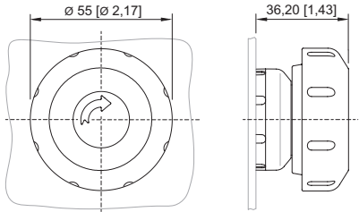
8602/3-015 Bouton d'arrêt rouge / jaune Tête de commande avec actionnement axial
