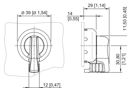
8602/3-727 Poignée rotative axiale, verrouillable Tête de commande avec actionnement axial
