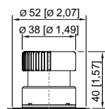
8003/...-010, 8003/...-012 Bouton d'arrêt Ø 38 mm
