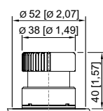
8003/...-010, 8003/...-012 Bouton d'arrêt Ø 38 mm
