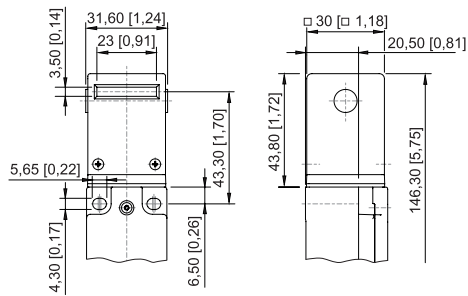
Interrupteur de sécurité 8060/2--AZ-60
