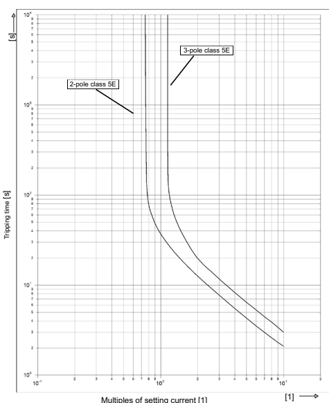
Courbe caractéristique de déclenchement 8510/132-05-335-301, Class 5E
