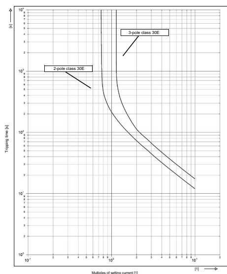
Courbe caractéristique de déclenchement 8510/132-05-335-301, Class 30E
