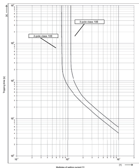
Courbe caractéristique de déclenchement 8510/132-05-335-301, Class 10E
