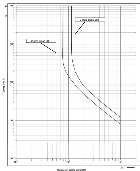
Courbe caractéristique de déclenchement 8510/132-05-335-301, Class 20E
