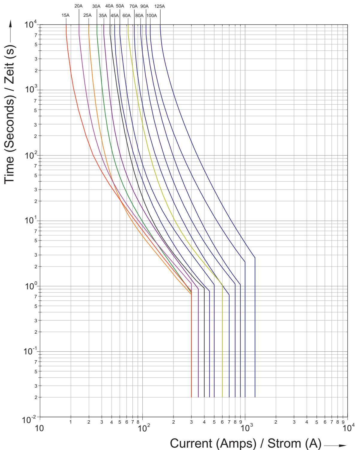
Courbes caractéristiques de déclenchement
