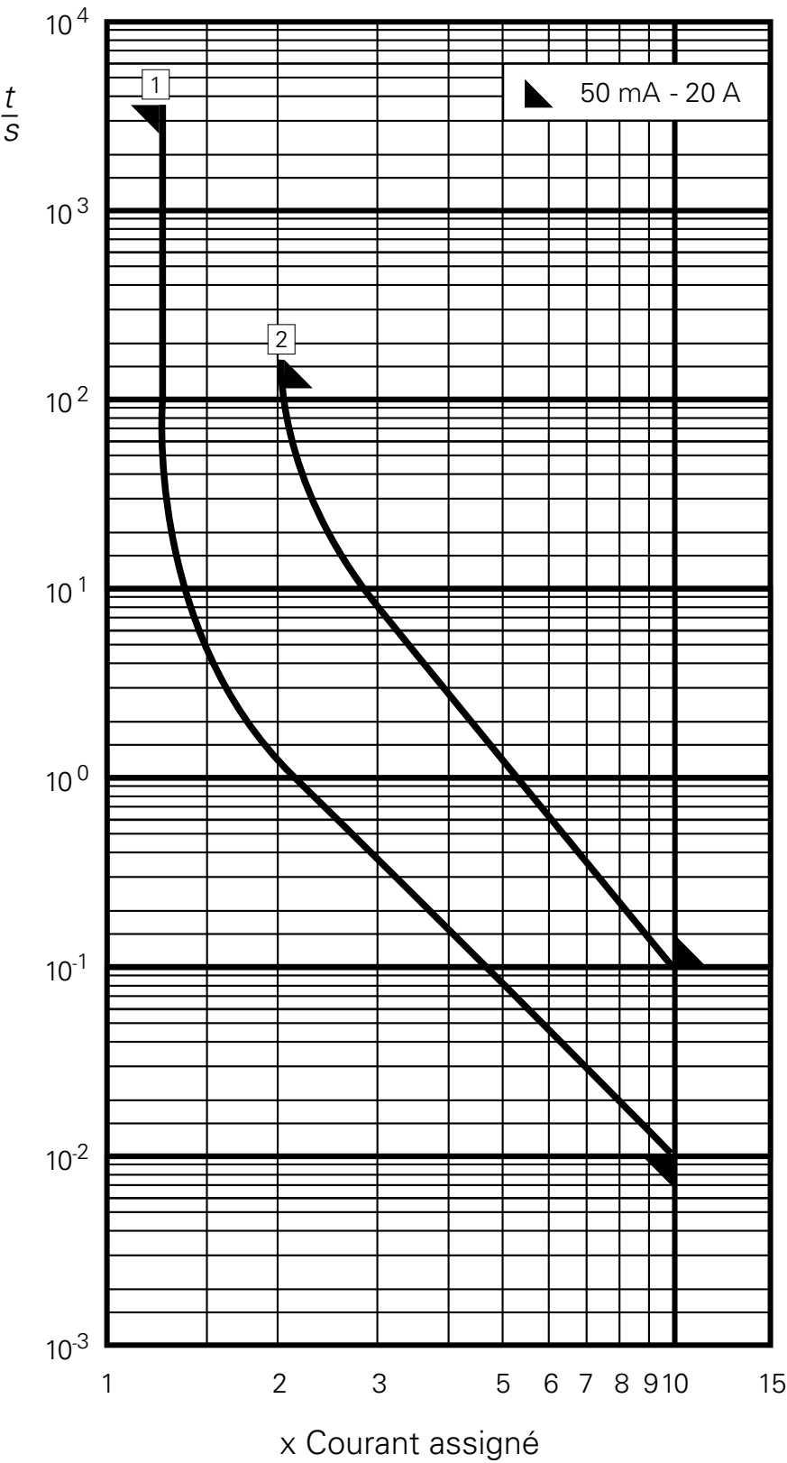
Courbe temps-courant 1 = durée de déclenchement minimal 2 = durée de déclenchement maximal
