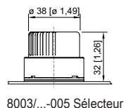
8003/...-005 Sélecteur
