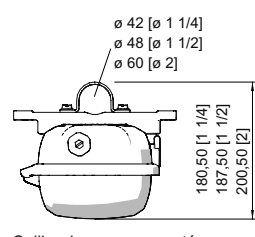
Collier de serrage monté sur support rail DIN
