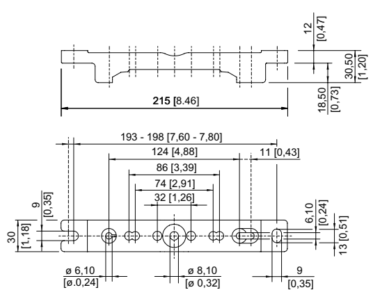
Support rail DIN
