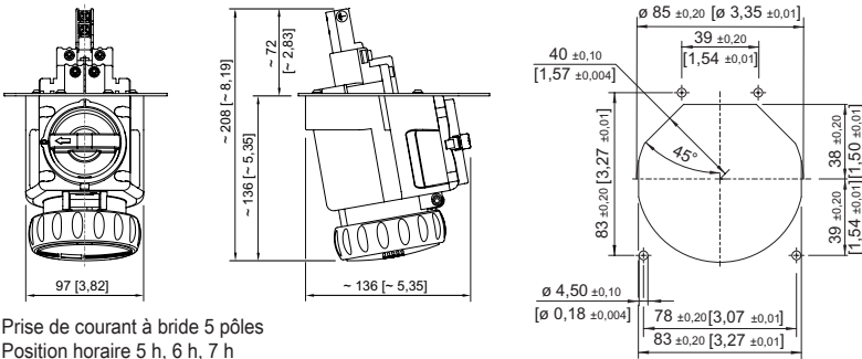
Prise de courant à bride 4/5 pôles Image d'ouverture
