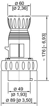
Fiche 4 pôles
