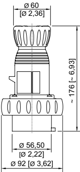
Fiche 5 pôles
