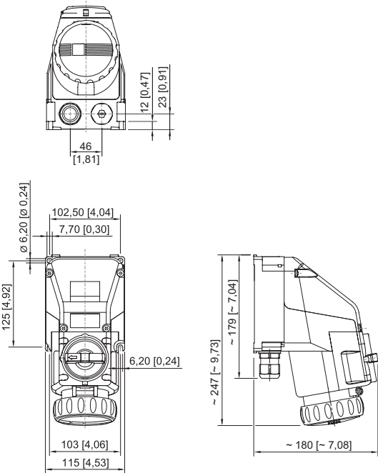
Prise murale 4 pôles / 5 pôles
