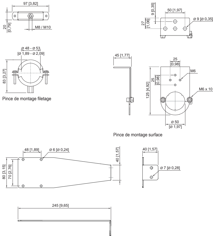
Plaqué de montage
