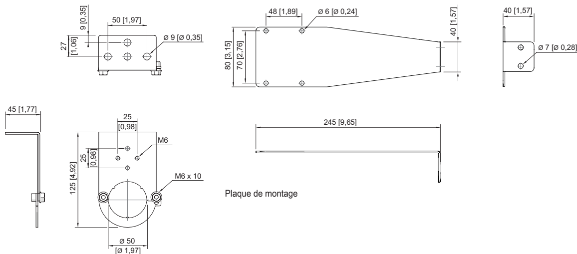
Pince de montage surface
