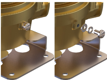
Tornillo de puesta a tierra con arandela elástica y arandela plana
