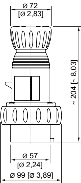
Enchufe de 4 polos
