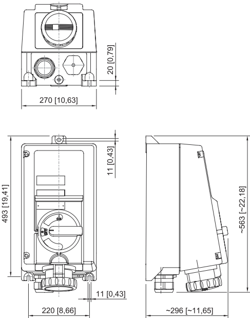
Toma de corriente de pared
